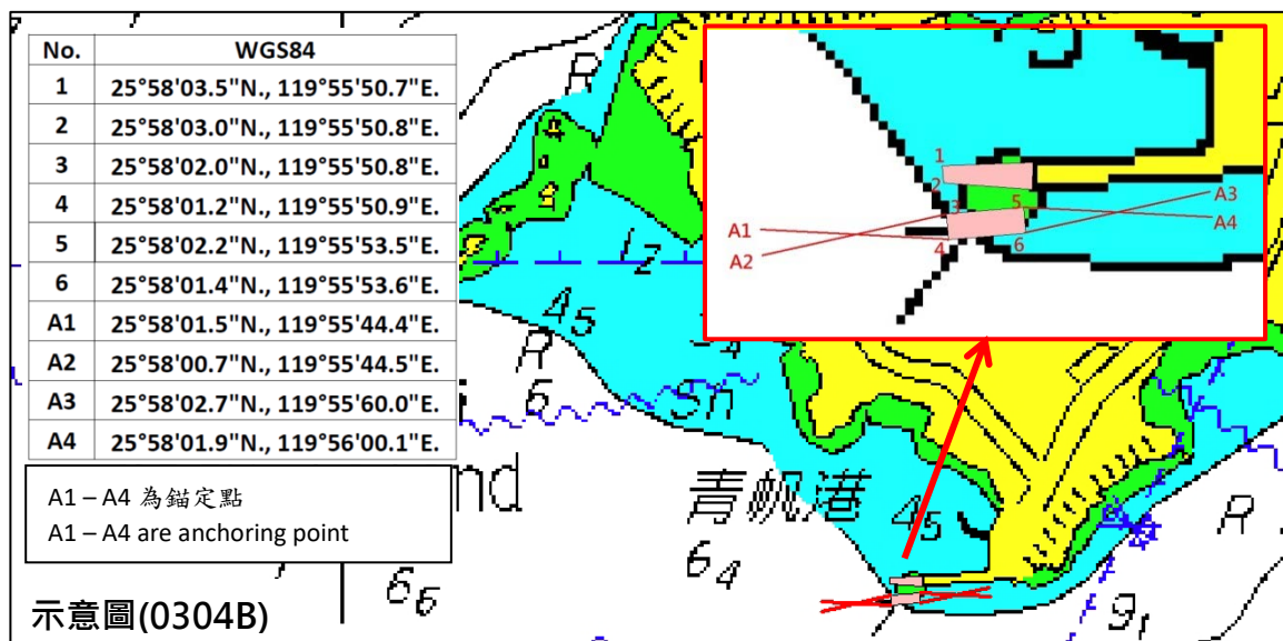
青帆碼頭區南防波堤堤頭拆除作業
