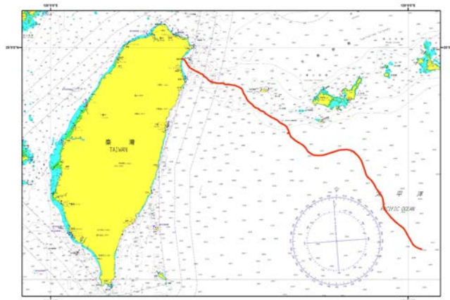
海纜佈放路線示意圖
